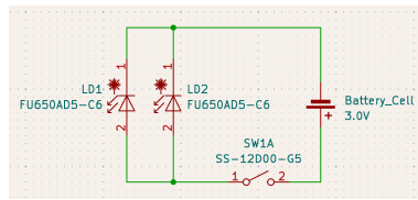
図 38 レーザー回路図
