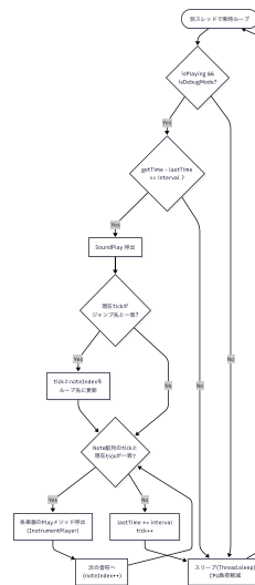
図 34 audioThread の処理ループおよび SoundPlay 関数のフローチャート
